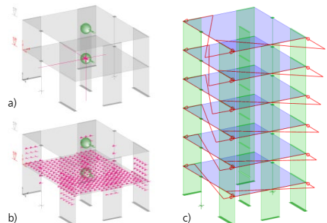
a) Ersatzlasten im selektierten Auswertungsraum
