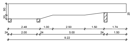
Schalplanausschnitt: mehrfach gevouteter Träger
