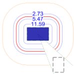
Erforderliche Durchstanzbewehrung je Rundschnitt an Rechteckstütze
