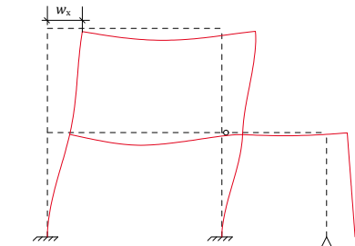
Nachweis Kopfverschiebungen
