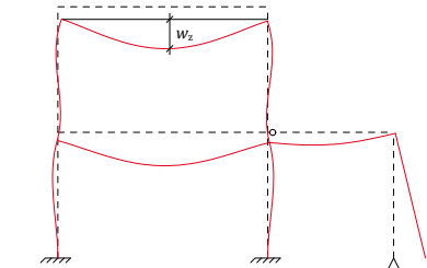
Nachweis Durchbiegung Einzelstäbe
