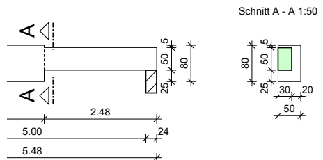
Schalplanausschnitt: Träger mit Querschnittsprung und Versatz
