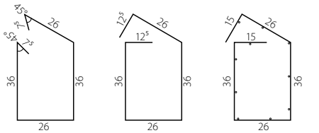
Biegeformen Rechteckbügel
